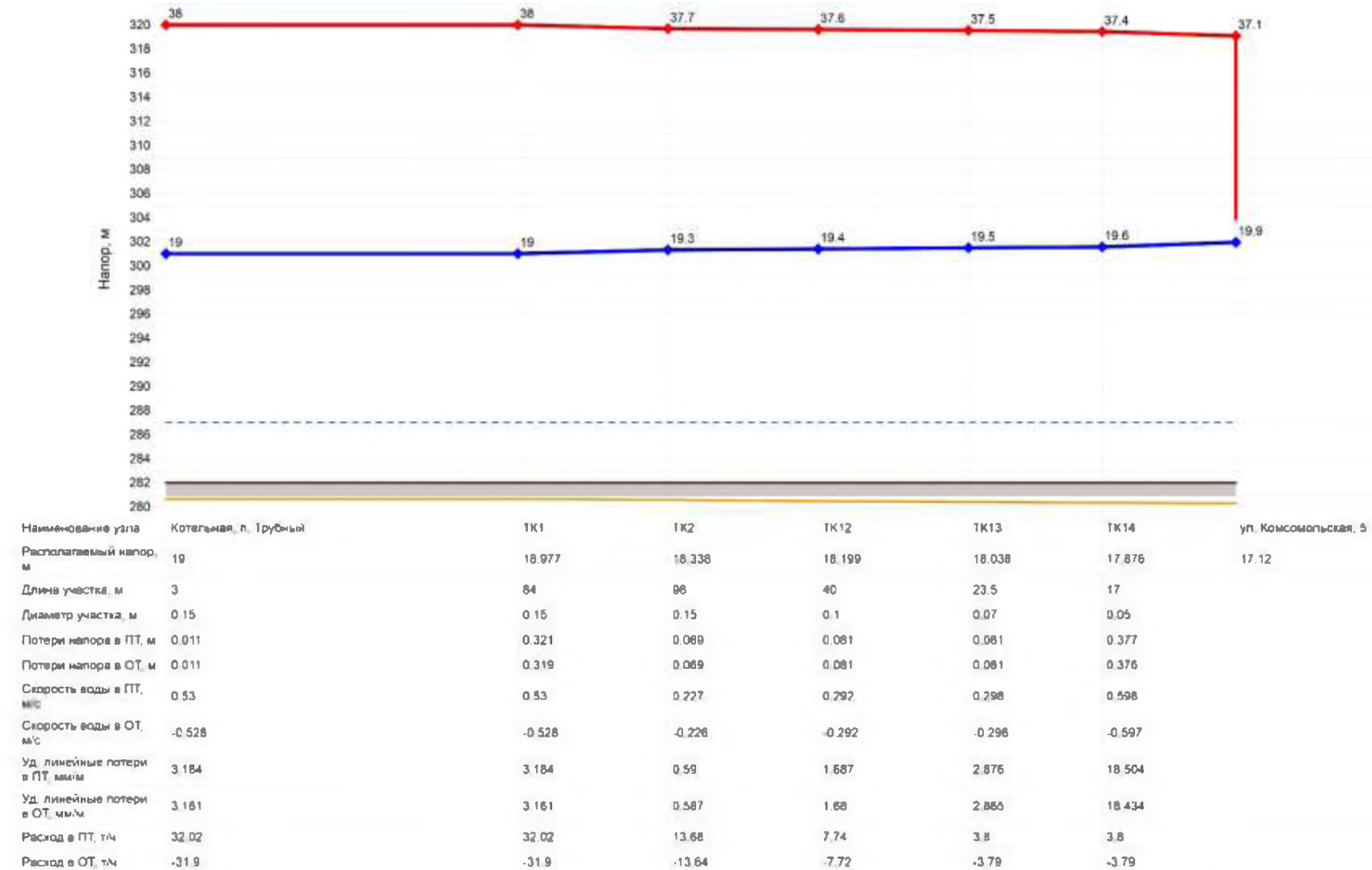
Рисунок 1.3.8.1. Пьезометрический график от Котельной, п. Трубный, ул. Верхняя, 19 до ул. Комсомольская, 5
