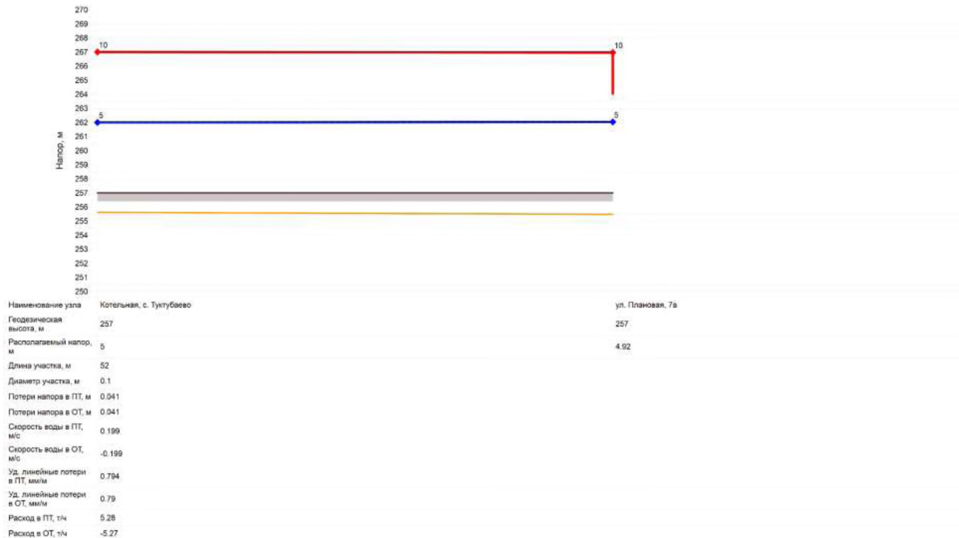
Рисунок 1.3.8.4. Пьезометрический график от Котельной, с. Туктубаево, ул. Плановая, 7 до ул. Плановая, 7а
