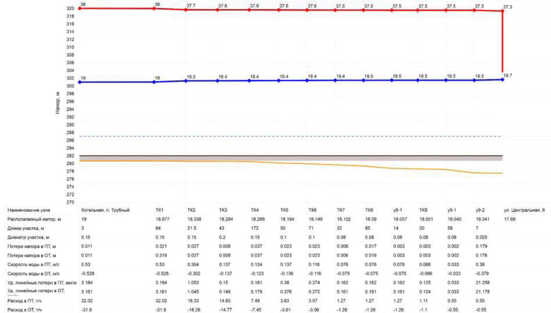
Рисунок 1.3.8.2. Пьезометрический график от Котельной, п. Трубный, ул. Верхняя, 19 до ул. Центральная, 6
