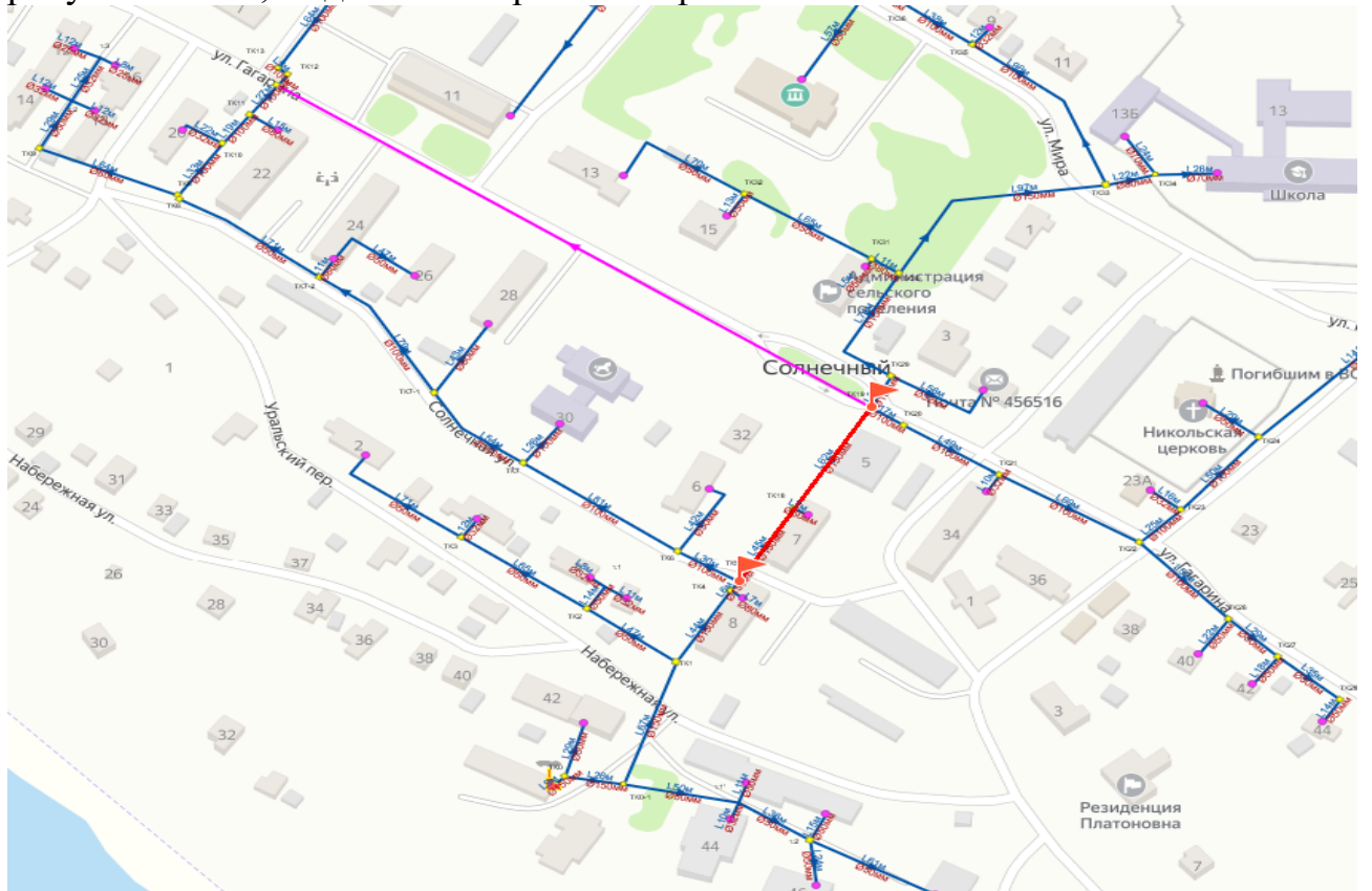
Рисунок 11.6.1. Сценарий развития аварии системы теплоснабжения
