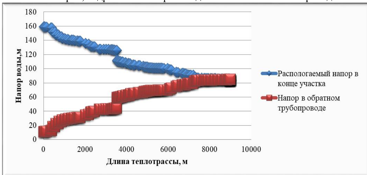
Рисунок 2.7 – Пьезометрический график тепловой сети центральной котельной по магистральному выводу
