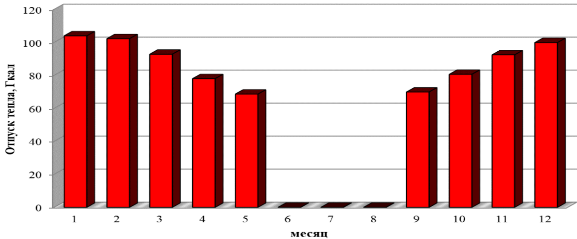
Рисунок 1.3 – Оптимальный температурный график отпуса тепловой энергии для школьной котельной
