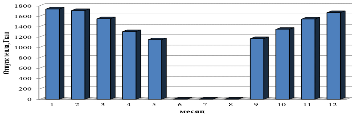
Рисунок 1.2 – Оптимальный температурный график отпуска тепловой энергии для центральной котельной
