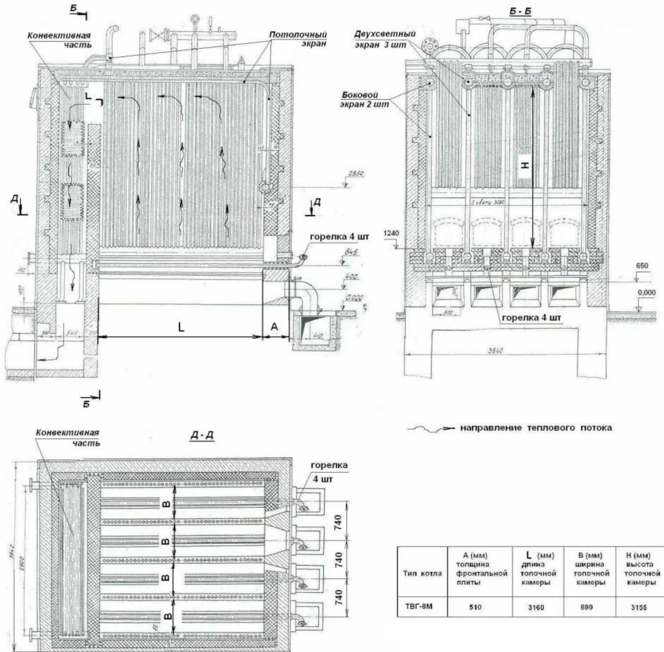
Рисунок 2.1 – Котел ТВГ-8М
