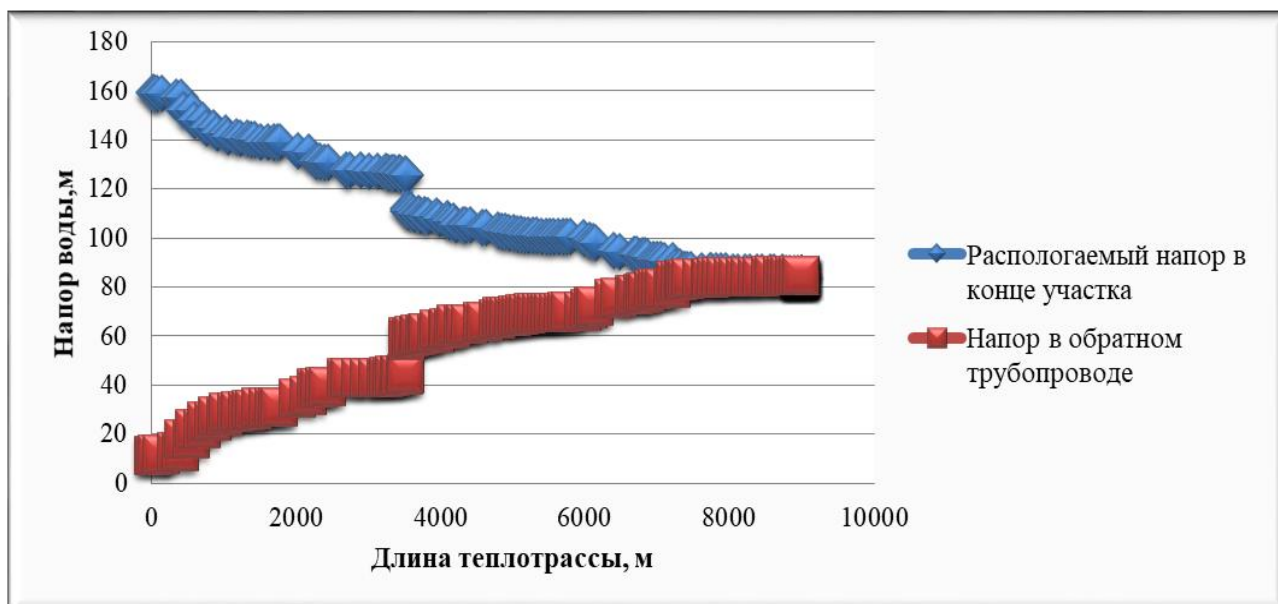
Рисунок 2.9 – Пьезометрический график тепловой сети центральной котельной по магистральному выводу Котельная ул. Лесная имеет один магистральный вывод на тепловые сети.
