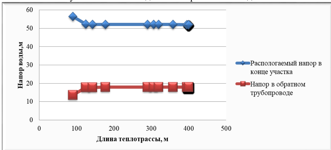
Рисунок 2.10 – Пьезометрический график тепловой сети котельной ул. Лесная по магистральному выводу
