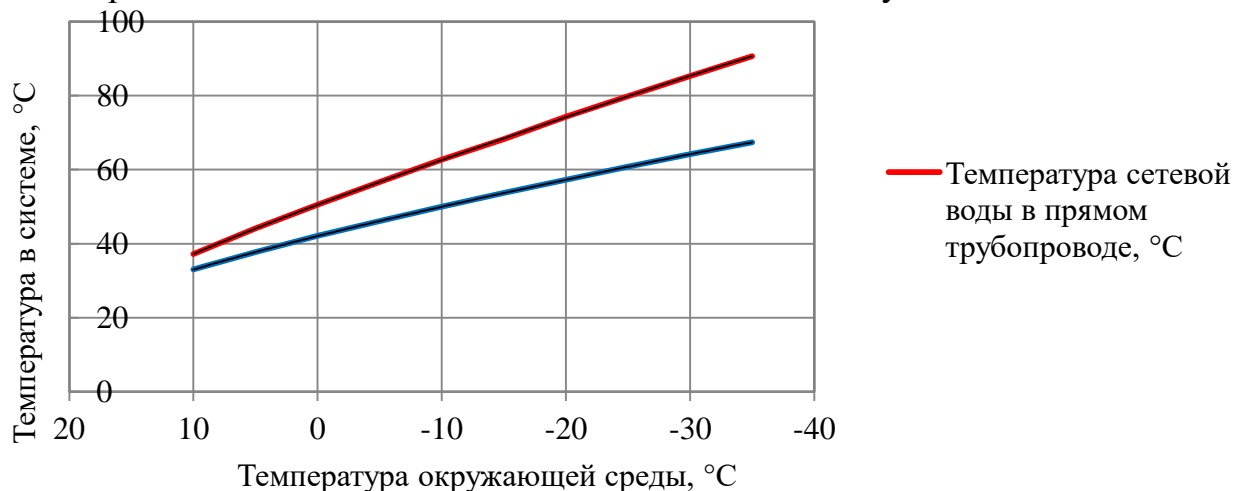
Рисунок 2.6 – График изменения температур теплоносителя
