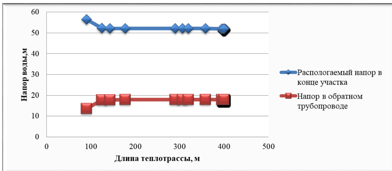
Рисунок 2.8 – Пьезометрический график тепловой сети котельной ул. Лесная по магистральному выводу
