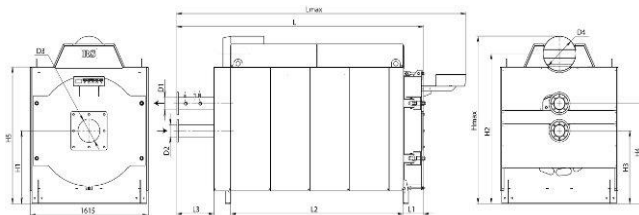
Рисунок 2.2 – Котел RS-D2000
