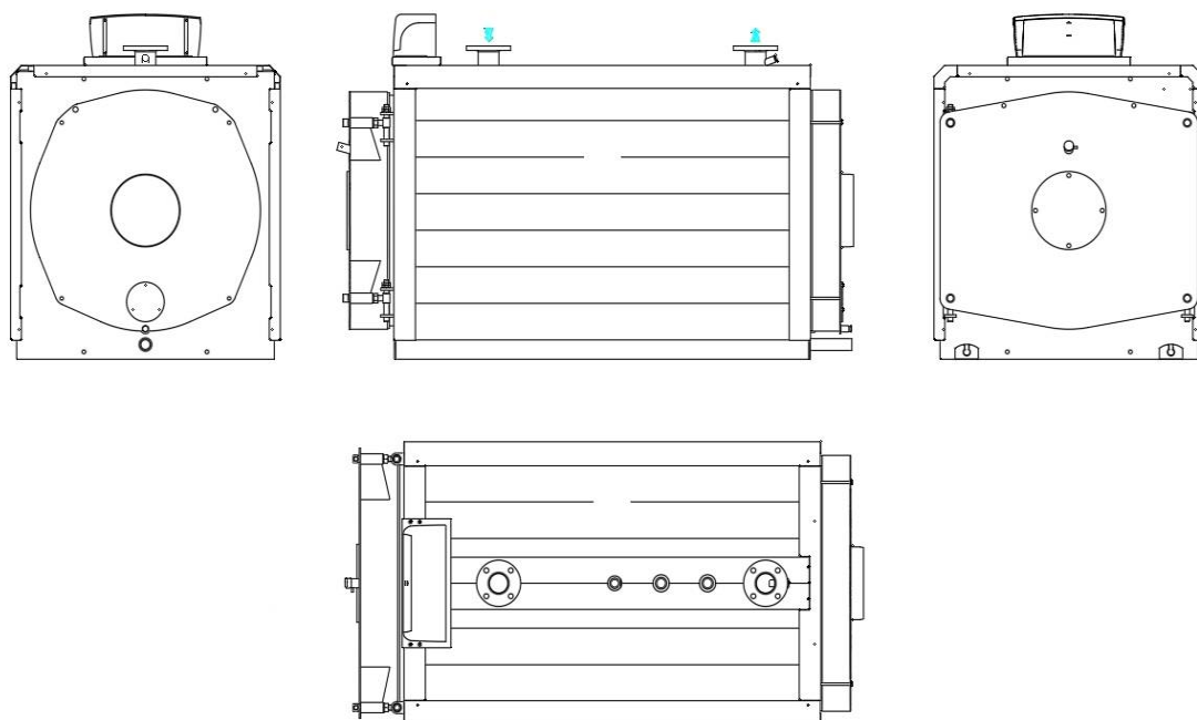
Рисунок 2.3 – Общий вид котлов ICI REX
