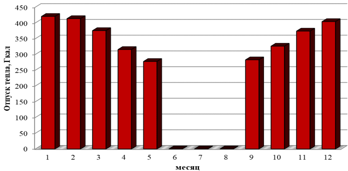
Рисунок 1.3 – Оптимальный температурный график отпуса тепловой энергии для котельной ул. Лесная
