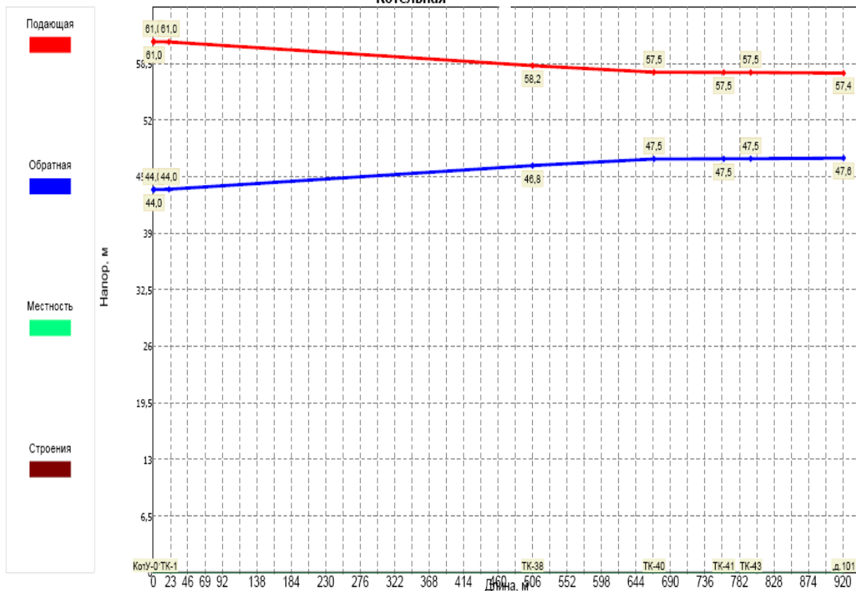
График падения напоров Котельная
