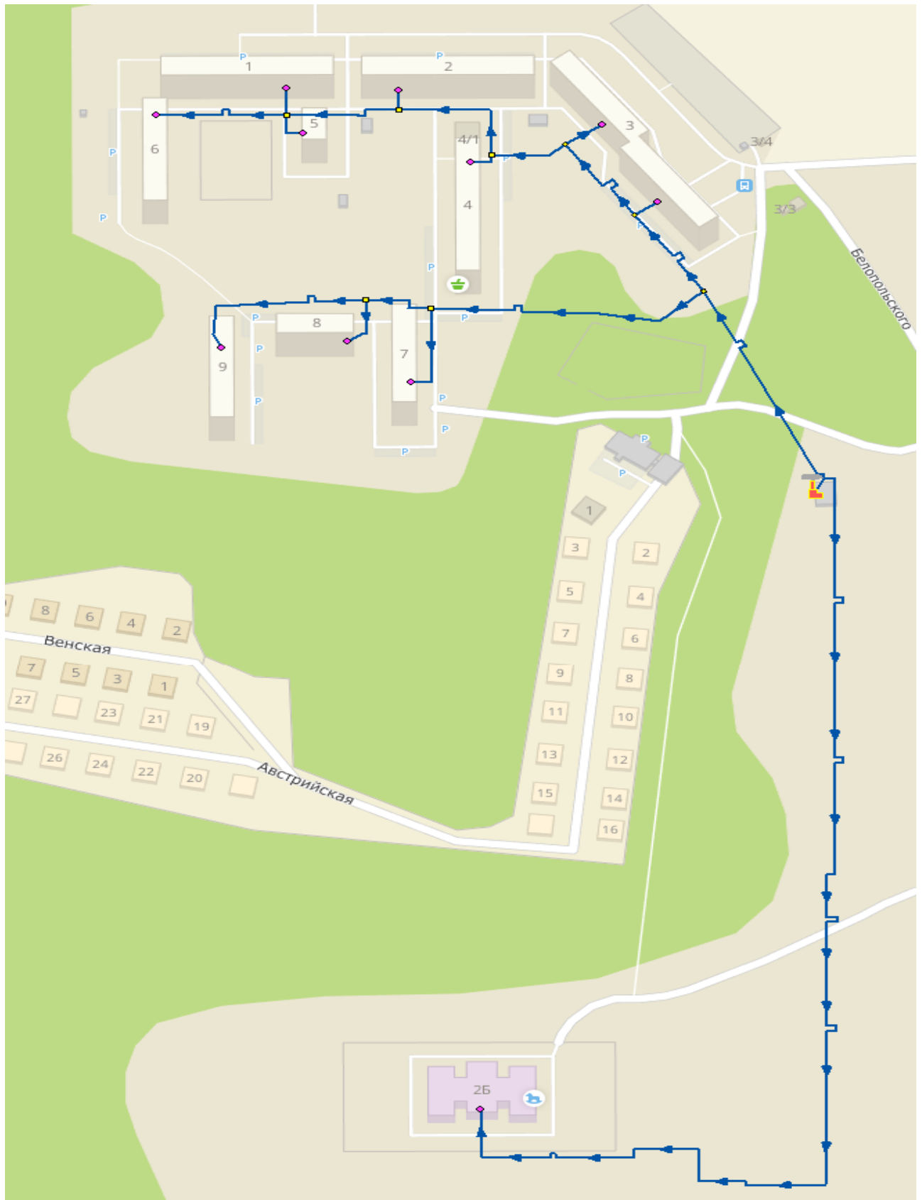
Рисунок 4-1. Схема сетей в контуре котельной «мкр. Звездный»
