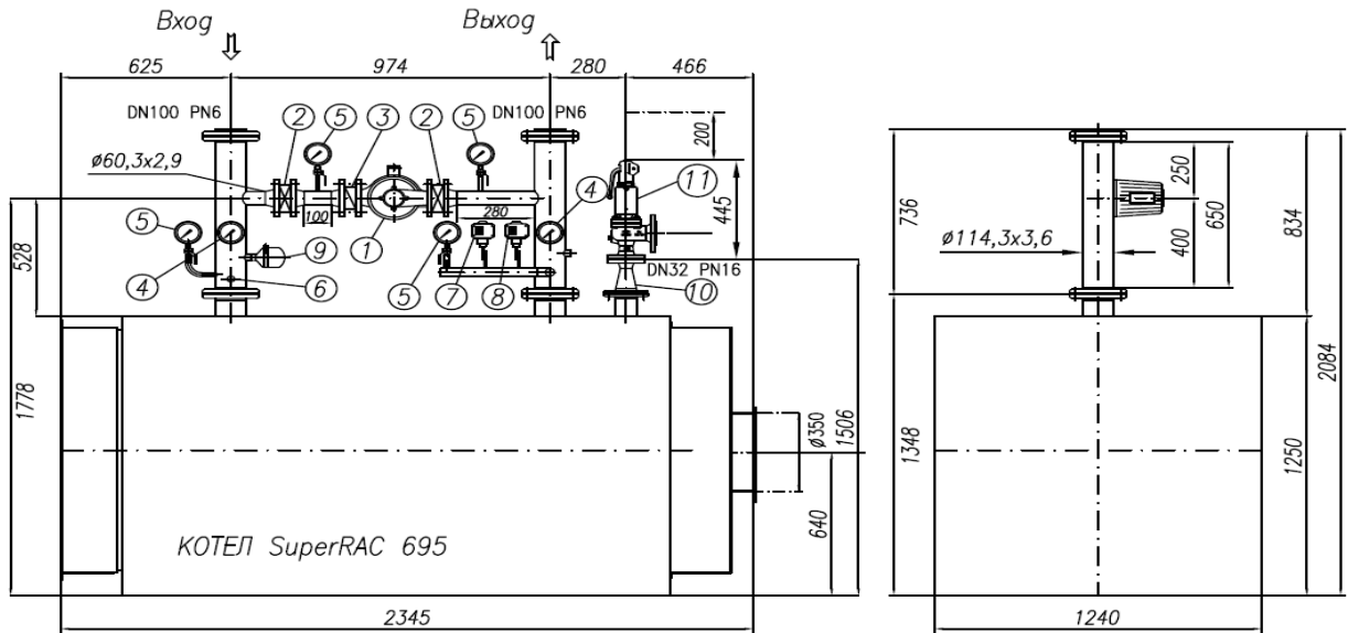
Рисунок 2.2.2-1 Котел SuperRac 695
