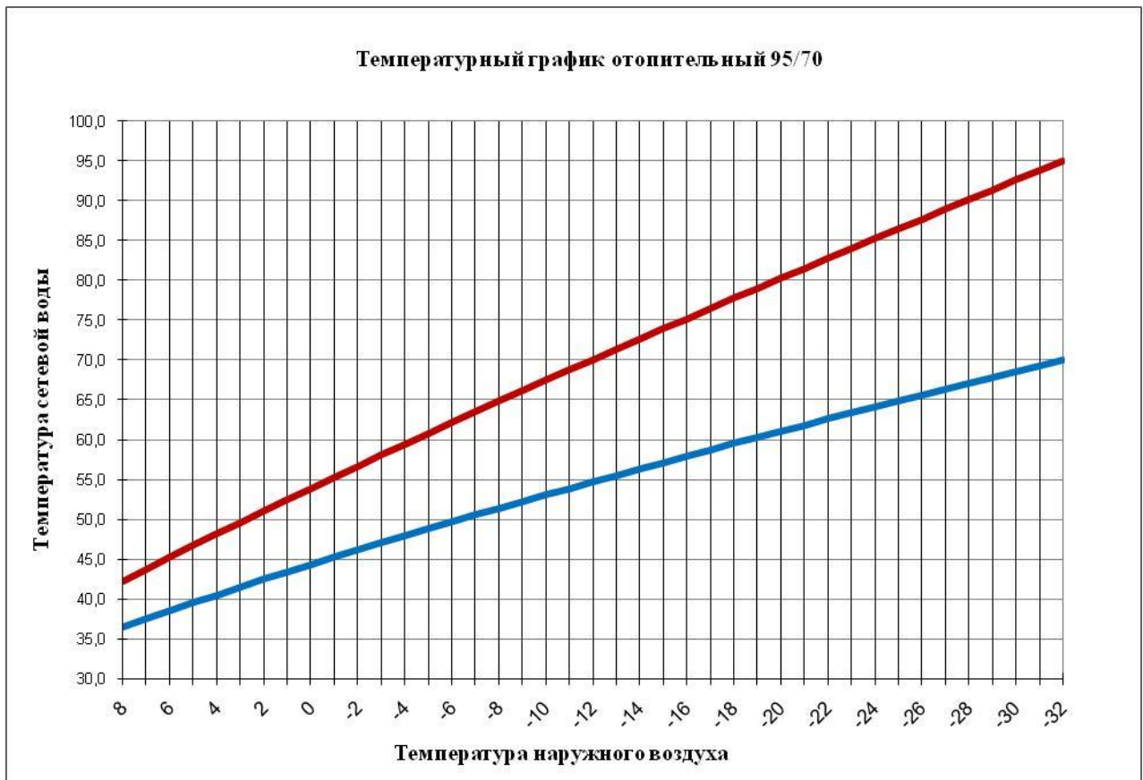
Рис. 2.7-1 Отопительный график качественного регулирования
