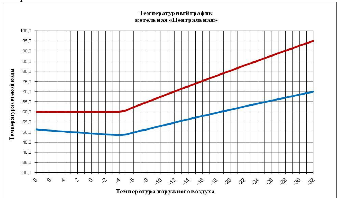
Рисунок 12 Предлагаемый температурный график Транспортабельная блочная котельная
