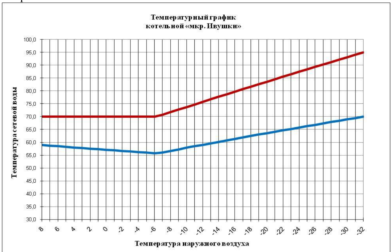
Рисунок 11 Предлагаемый температурный график «мкр. Ивушки»
