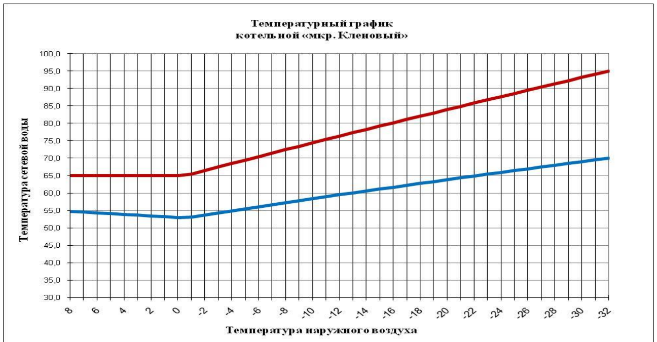
Рис. 2.7.2 – 1 Предлагаемый температурный график «мкр. Кленовый»
