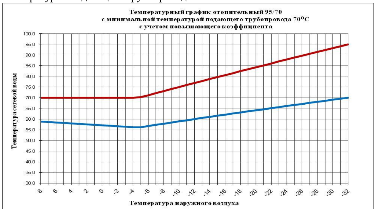
Рис. 2.7-3 График качественного регулирования 95/70 с минимальной температурой подающего трубопровода 70^{\circ}\text{C} с учетом повышающего коэффициента
