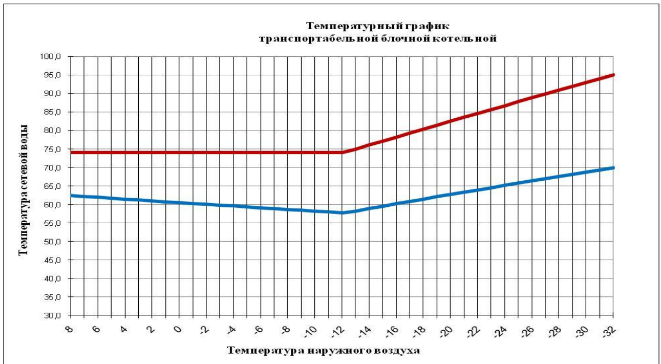
Рис. 2.7.5 – 1 Температурный график транспортабельной блочной котельной
