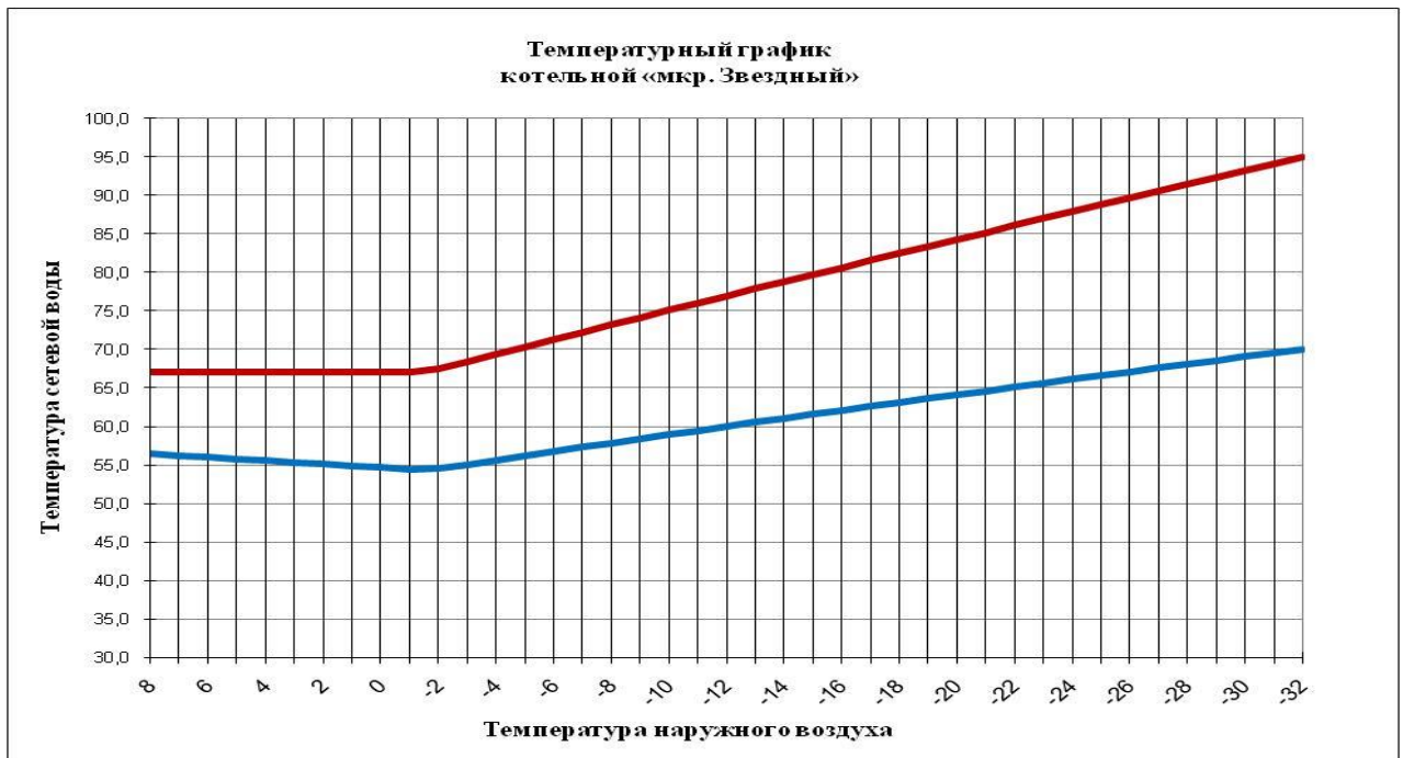
Рис. 2.7.1 – 1 Предлагаемый температурный график «мкр. Звездный»
