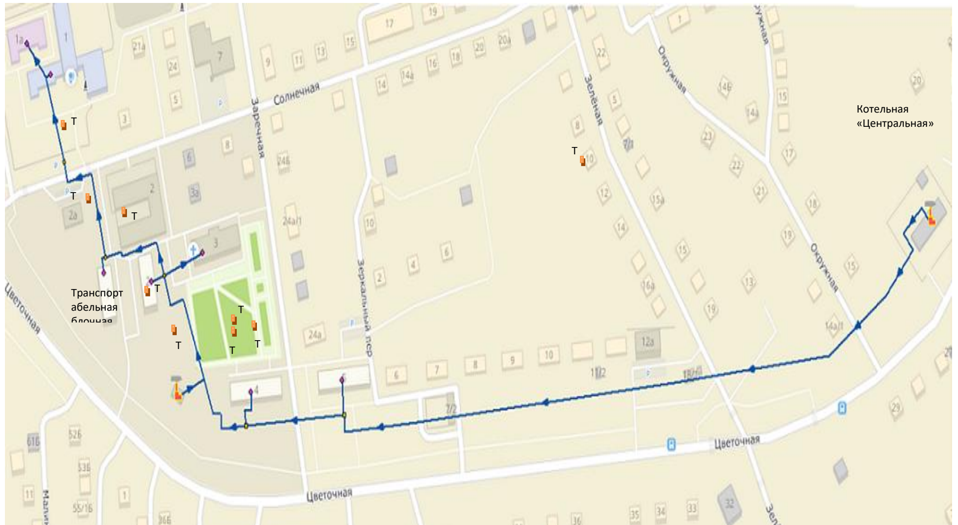
Рисунок 8 Схема тепловых сетей в контуре Транспортной блокной котельной с обозначением тепловых камер
