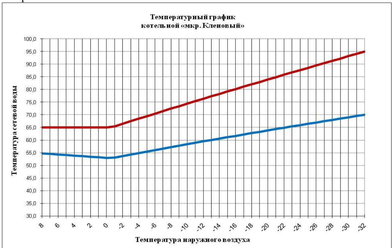
Рисунок 10 Предлагаемый температурный график «мкр. Кленовый»
