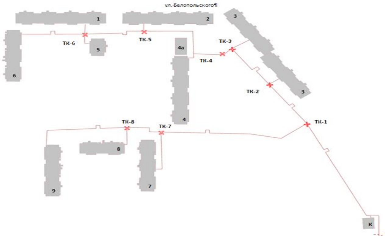
Рисунок 4-2. Схема северной части тепловых сетей в контуре котельной «мкр. Звездный» с обозначением тепловых камер
