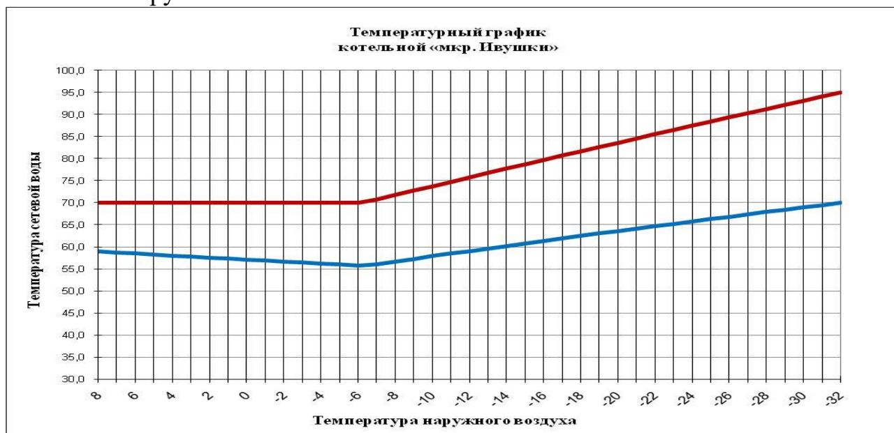
Рис. 2.7.3 – 1 Предлагаемый температурный график «мкр. Ивушки»
