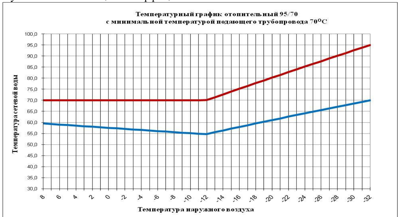
Рис. 2.7-2 График качественного регулирования 95/70 с минимальной температурой подающего трубопровода 70^{\circ}\text{C}
