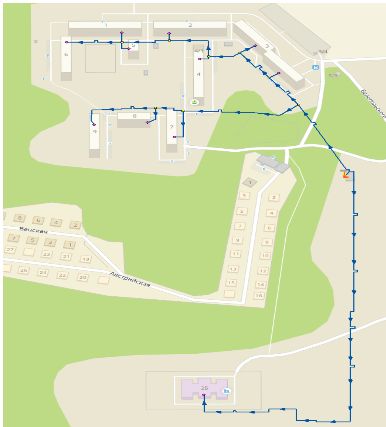
Рисунок 4 Схема сетей в контуре котельной «мкр. Звездный»
