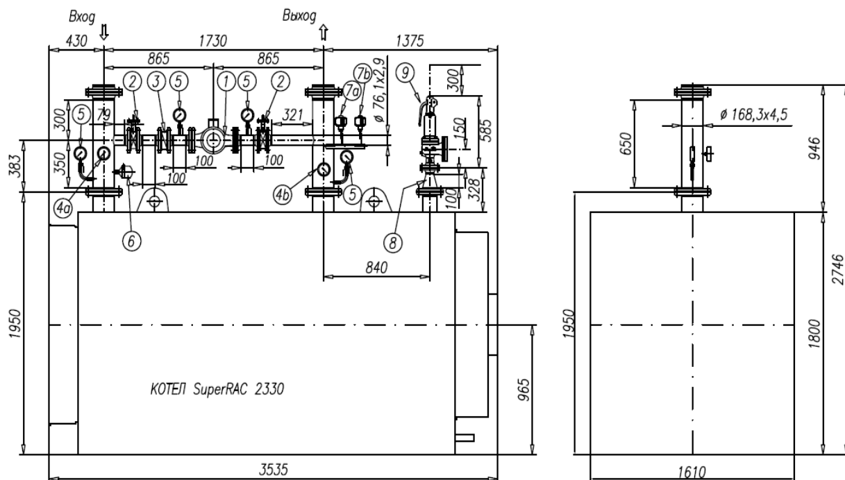
Рисунок 2.2.5-1 Котел SuperRac 2330
