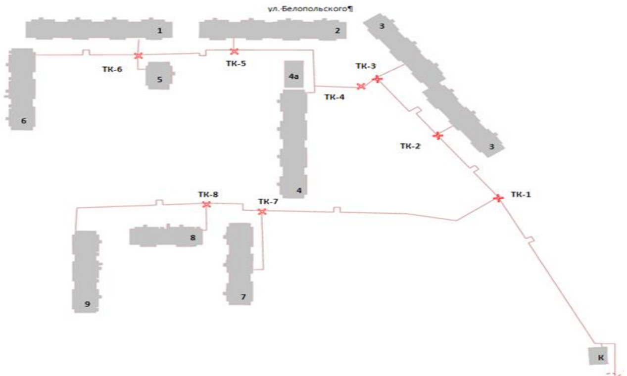
Рисунок 5 Схема северной части тепловых сетей в контуре котельной «мкр. Звездный» с обозначением тепловых камер
